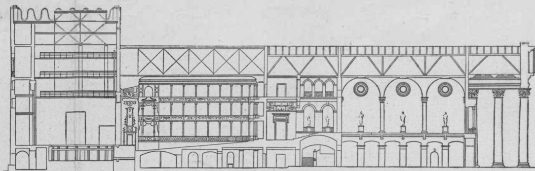
Разрез
