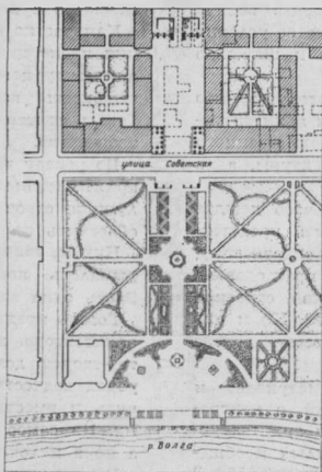
Схема генерального плана
